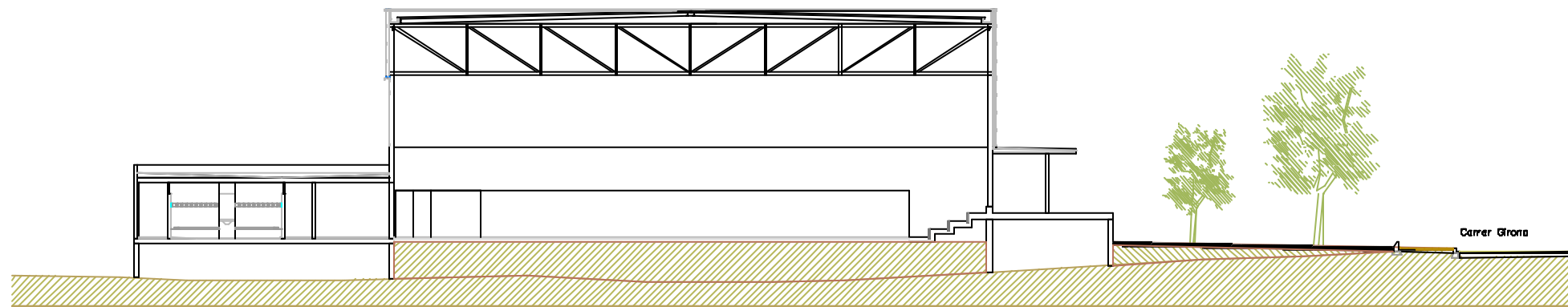
SECCIÓ TRANSVERSAL
